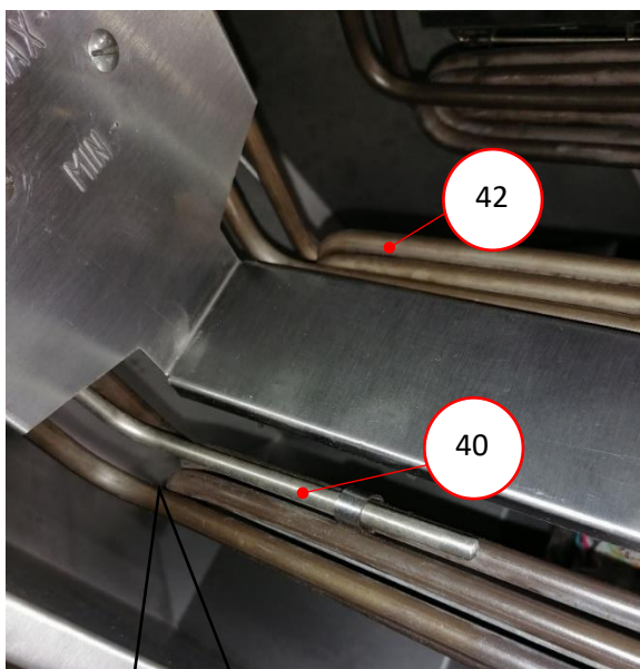
Датчик температуры (датчик температуры ТЭНа)
