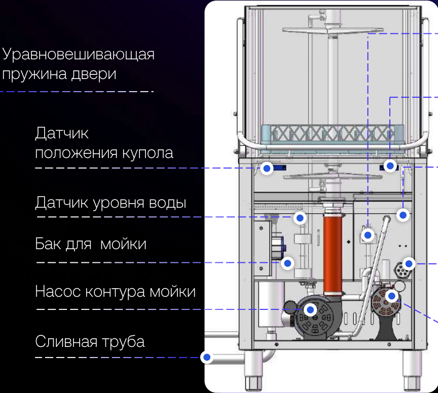
Вид спереди
